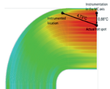
Calcul de point chaud
